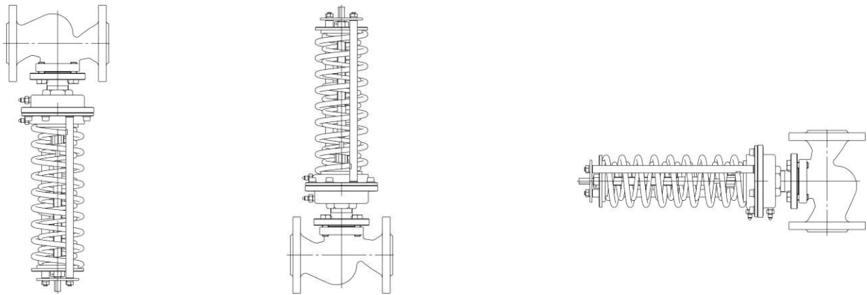
Рисунок А.3-Монтажные положения регулятора на трубопроводе при температуре среды до 100 °С (Прямолинейные участки до и после регулятора не требуются)
