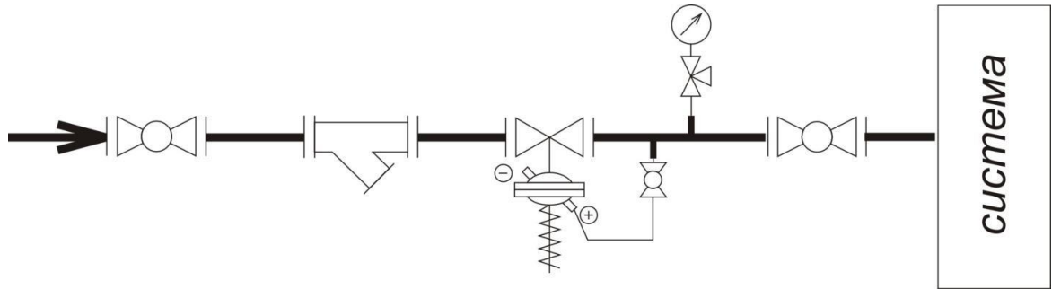
Регулятор давления «после себя» Рисунок А.2-Схема подключения регулятора
